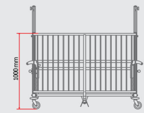
najniższa pozycja poręczy bocznej 1000 mm
