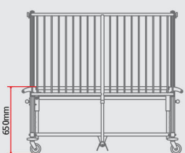
najniższa pozycja leża 650 mm
